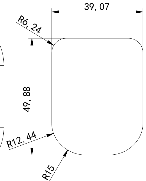
布料冲孔尺寸图
